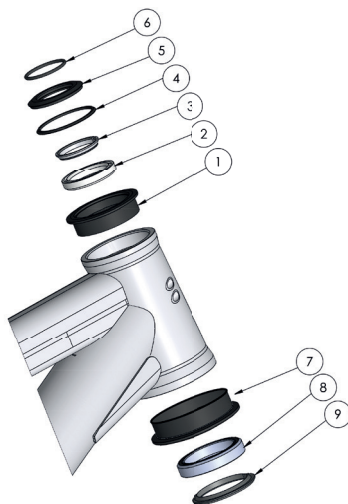
Abb.: Steuersatzaufbau
