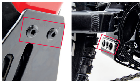
Abb.: Befestigungspunkte für das Skidplate
