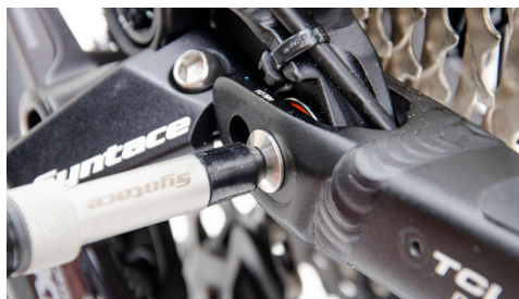
Abb.: Abschmierbare Lagerstelle am Horstlink
