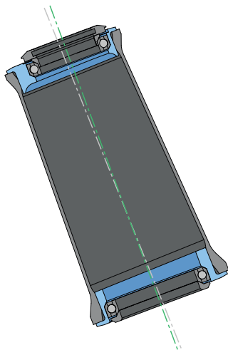
Steuerrohrwinkel -1,5^\circ
