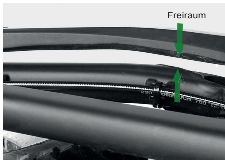
Abb.: Freiraum zwischen Kettenführung und Kettenstreben
