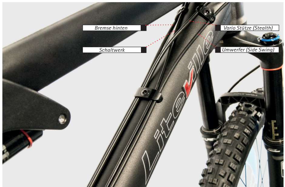
Abb. zeigt: Beispielhaft 2x11 Antriebseinheit, Bremseinheit und Vario-Stütze am Unterrohr
